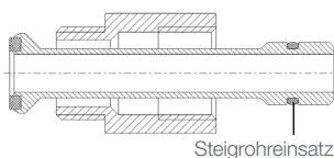
Verlängerung ½"
